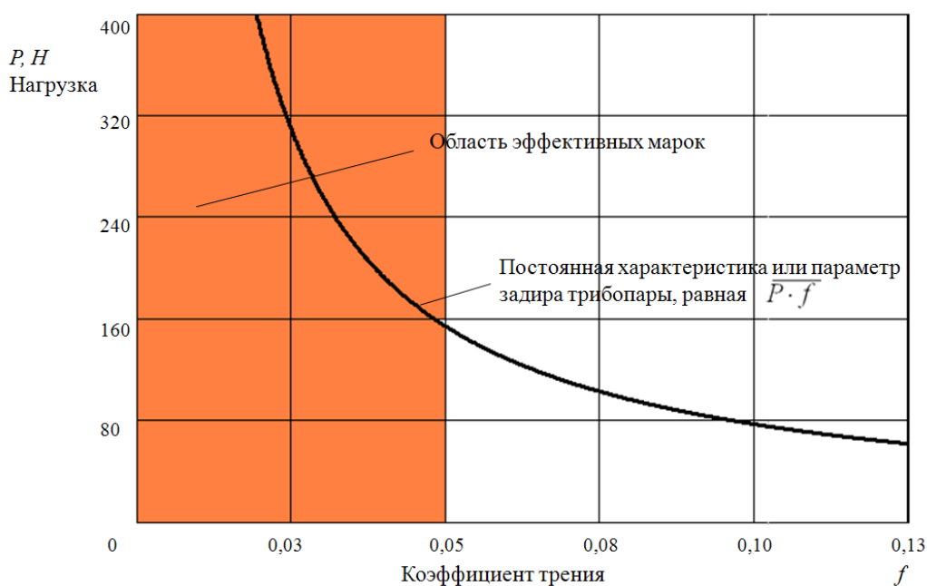
Рисунок 2 – Область эффективных марок наноматериалов
